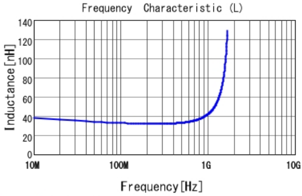
LQG15HZ33NJ02 L
