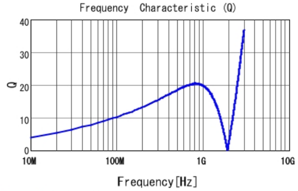
LQG15HZ33NJ02 Q
