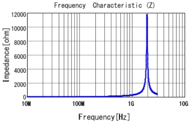
LQG15HZ33NJ02 |Z|
