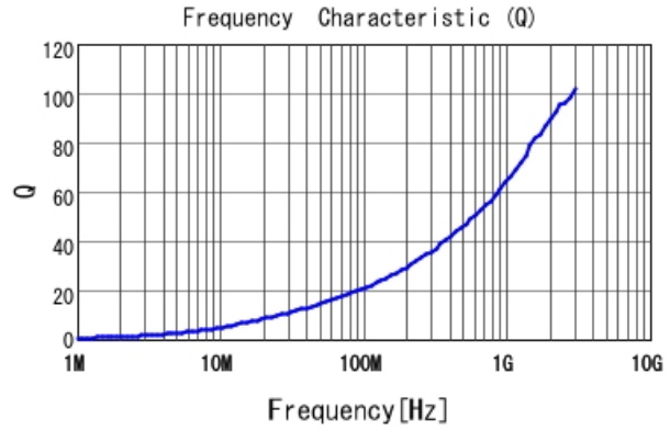
LQW15AN4N7D8Z Q
