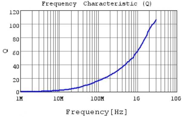
LQW15AN1N7C8Z Q
