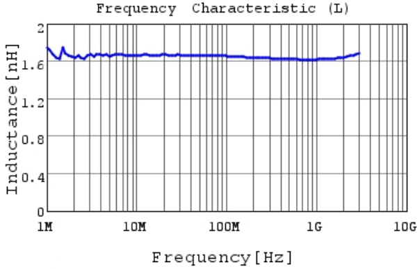
LQW15AN1N7C8Z L
