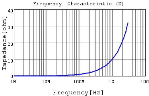
LQW15AN1N7C8Z |Z|
