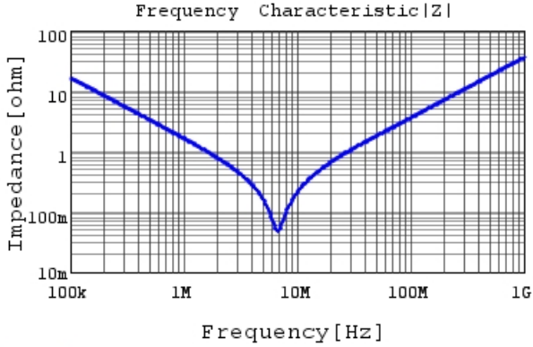
RDER72E104K2M1H03A |Z| DCOV, 25degC
