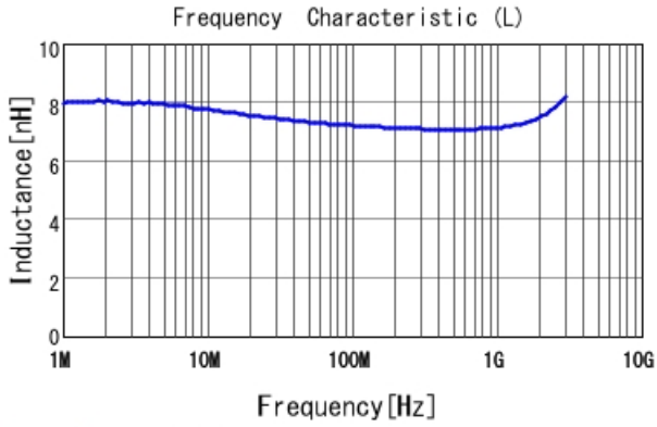
LQW15AN7N3G80 L
