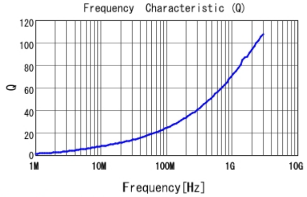
LQW15AN7N3G80 Q
