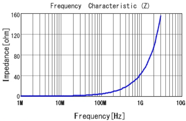
LQW15AN7N3G80 |Z|
