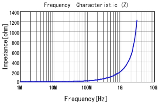
LQW15AN33NJ80 |Z|
