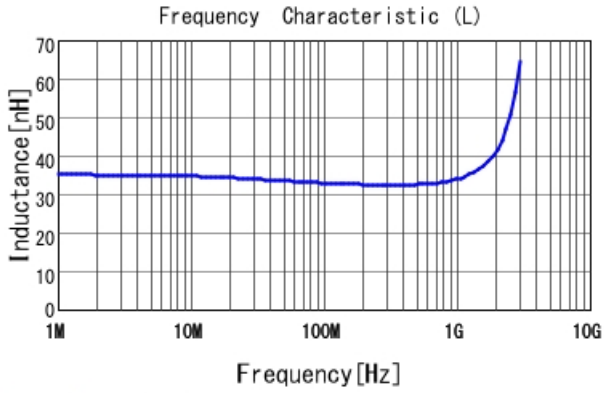
LQW15AN33NJ80 L
