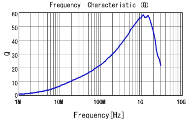
LQW15AN33NJ80 Q
