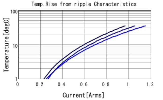
GRM1555C2A390JA01 Temp. rise — 500MHz — 700I
