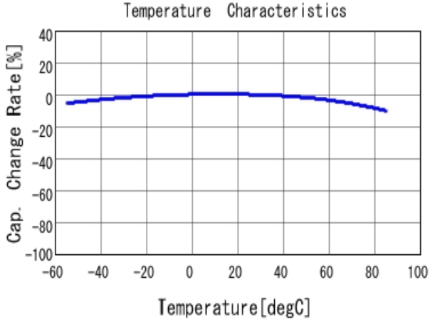
■ GRM155R61A154KE19 C-Temp. capchange, DCO. 0V, ACO. 5V rm
