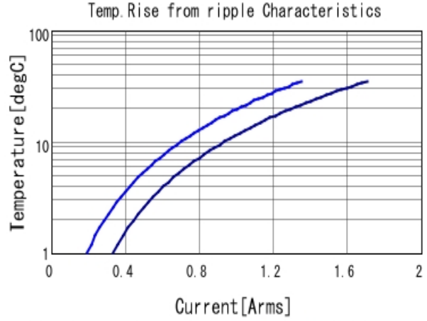
GRM155R61A154KE19 Temp. rise ■ 500kHz ■ 1MHz
