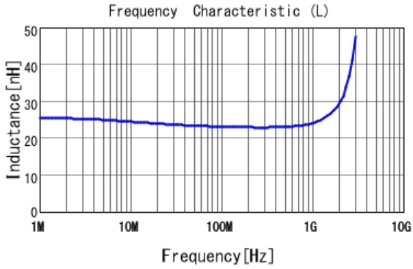
LQW18AN23NJ8Z L
