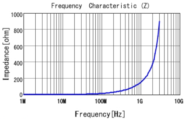
LQW18AN23NJ8Z |Z|
