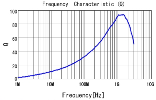
LQW18AN23NJ8Z Q
