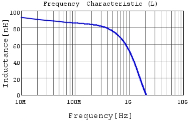
LQW18CNR10K0Z L
