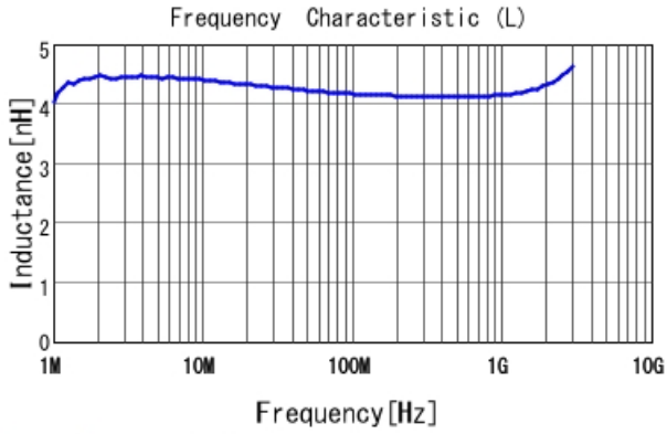
LQW15AN4N1G8Z L
