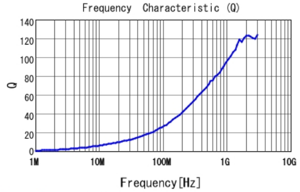
LQW15AN4N1G8Z Q
