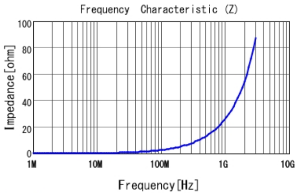
LQW15AN4N1G8Z |Z|
