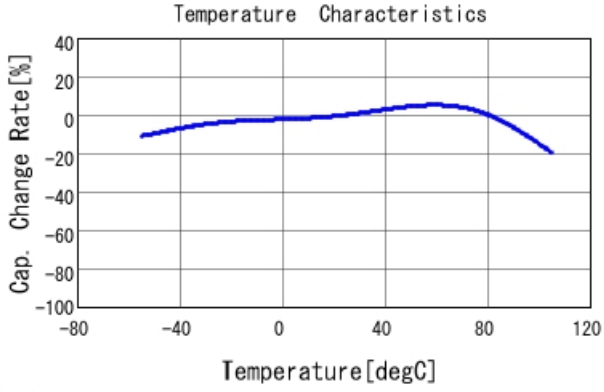
■ GRM32EC81A476ME19 C-Temp. capchange, DCO. 0V, ACO. 5Vrm
