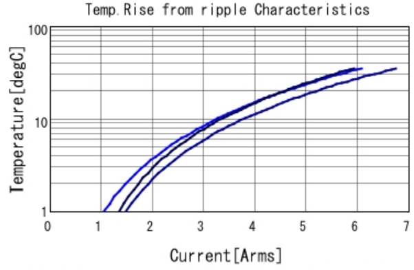
GRM32EC81A476ME19 Temp. rise ■ 60kHz ■ 300kHz ■ 600kHz
