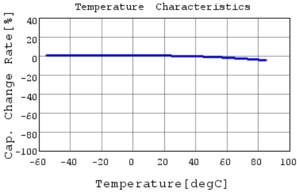
GRM033R61E681KA01 C-Temp. capchange, DCO.OV,
