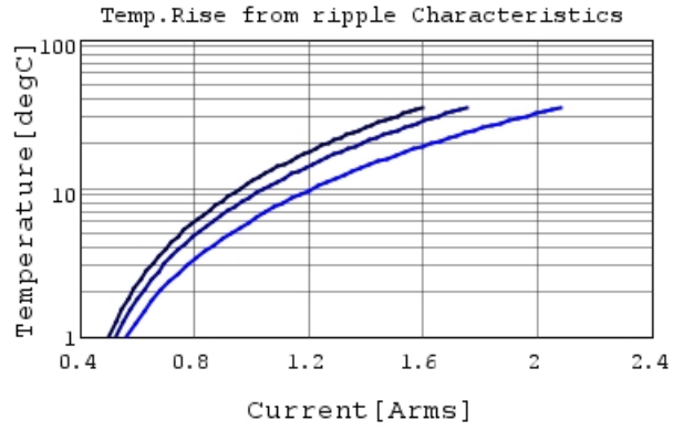
GQM1875C2E101GB12 Temp.rise — 300MHz —
