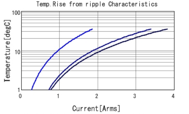
GRM188R61E105KAAD Temp. rise — 100kHz — 500
