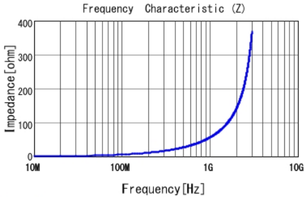
LQG15HH9N1G02 |Z|
