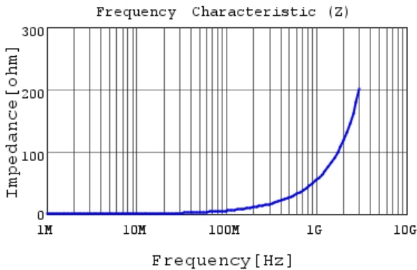
LQW15AN8N6G80 |Z|
