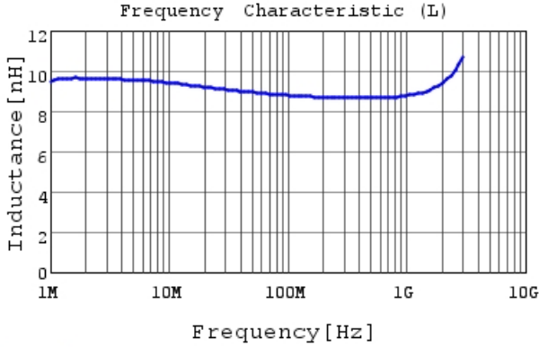
LQW15AN8N6G80 L
