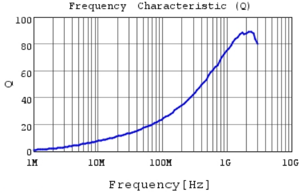
LQW15AN8N6G80 Q
