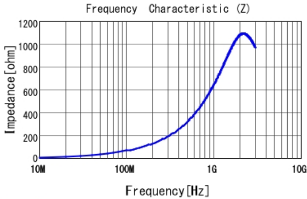
LQW15CAR11J00 |Z|
