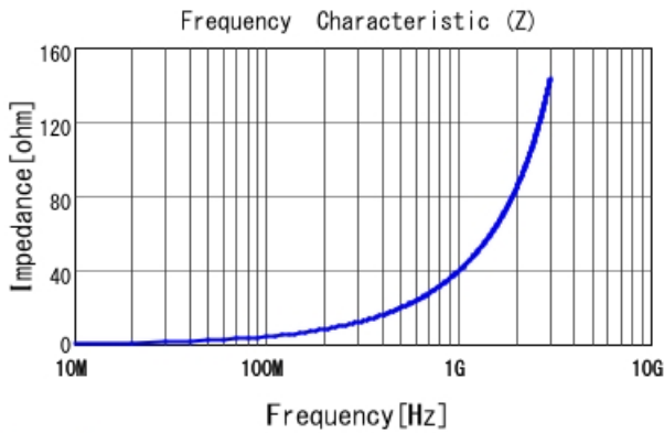
LQP03TN6N2H02 |Z|
