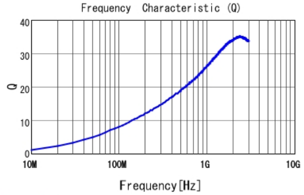
LQP03TN6N2H02 Q
