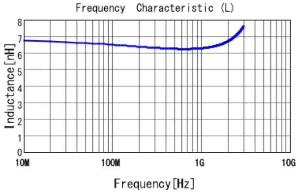
LQP03TN6N2H02 L
