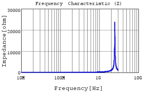
LQG15WH30NG02 |Z|
