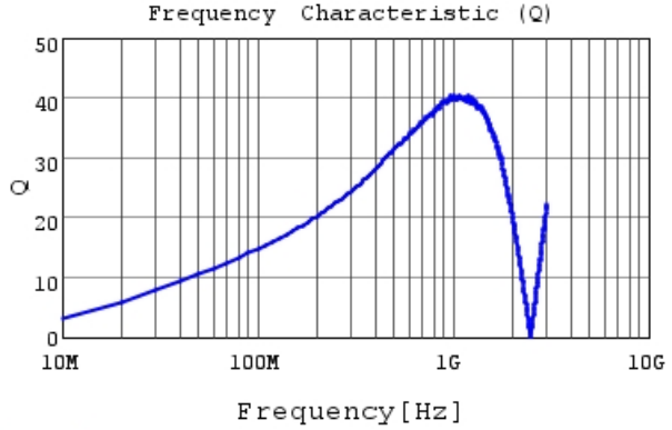
LQG15WH30NG02 Q
