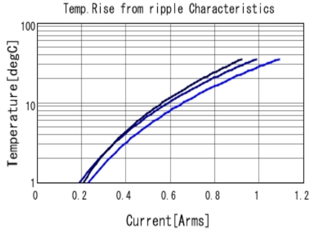
GRM1555C1H220JA01 Temp. rise ■ 500MHz ■ 700MHz ■ 1GHz
