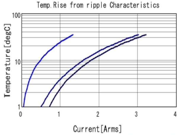
GRM155R61C474KE01 Temp. rise ■ 200kHz ■ 500kHz ■ 1MHz
