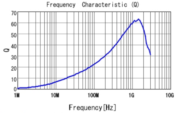
LQW15AN27NJ8Z Q
