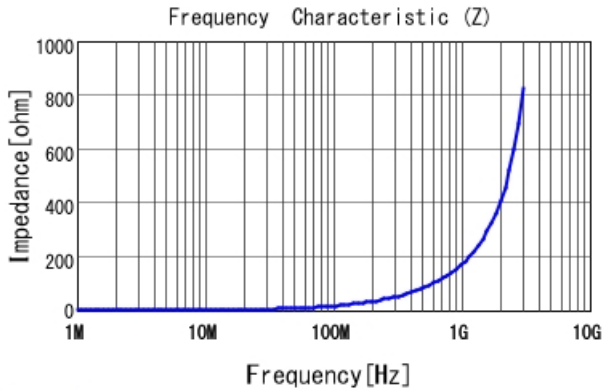
LQW15AN27NJ8Z |Z|
