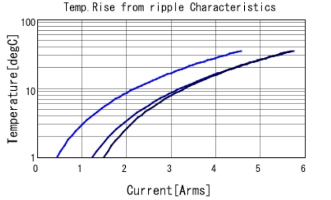
GRT21BR60J226ME13 Temp. rise — 80kHz — 400kHz
