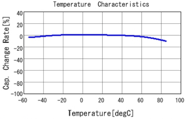
GRT21BR60J226ME13 C-Temp. capchange, DCO. 0V, ACO. 5
