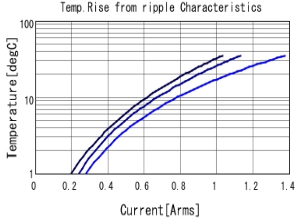
GRM1555C1H510JA01 Temp. rise ■ 200MHz ■ 500MHz ■ 700M
