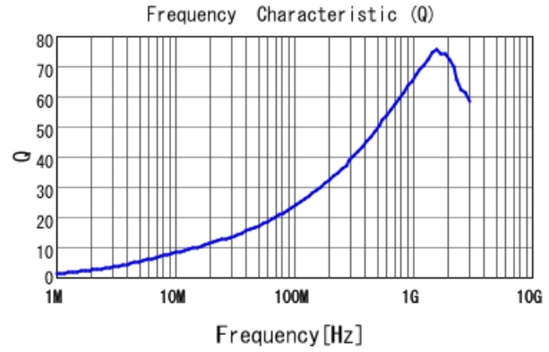
LQW15AN13NJ80 Q
