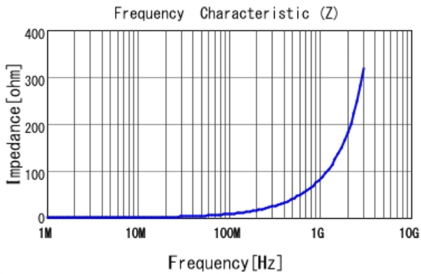
LQW15AN13NJ80 |Z|
