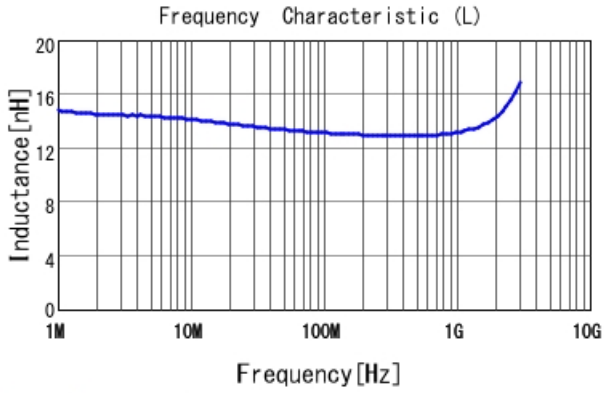
LQW15AN13NJ80 L
