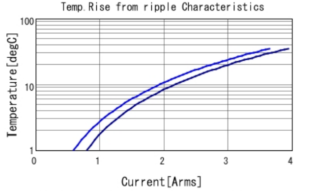
GRM188R61A225KE34 Temp. rise — 500kHz — 1MHz
