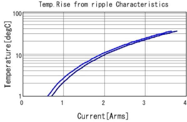
GRM188C71C225KE11 Temp. rise ■ 500kHz ■ 1MHz
