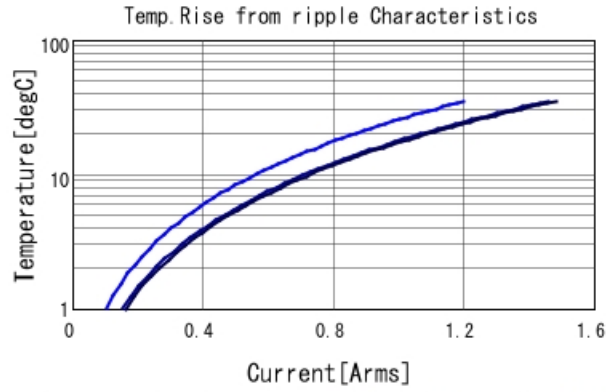
GCJ188R72A104MA01 Temp. rise ■ 400kHz ■ 800kHz ■ 1MHz
