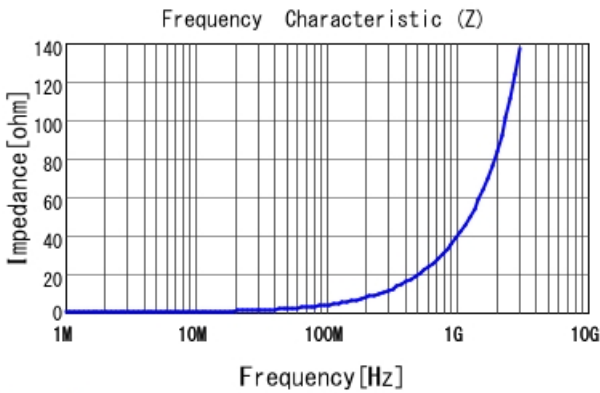
LQW15AN6N3G8Z |Z|
