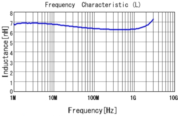
LQW15AN6N3G8Z L
