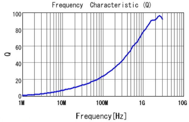
LQW15AN6N3G8Z Q
