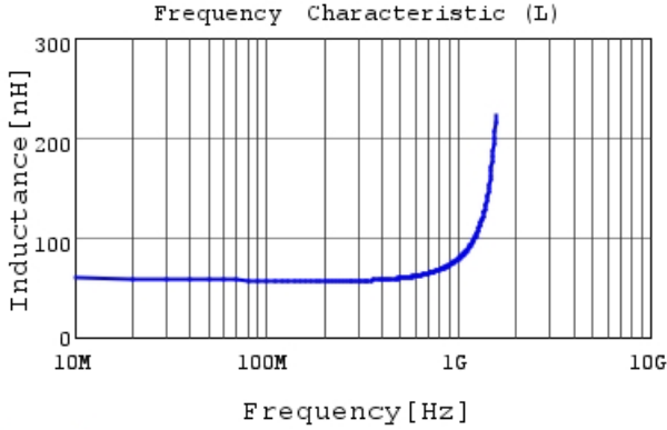
LQG15WH56NG02 L
