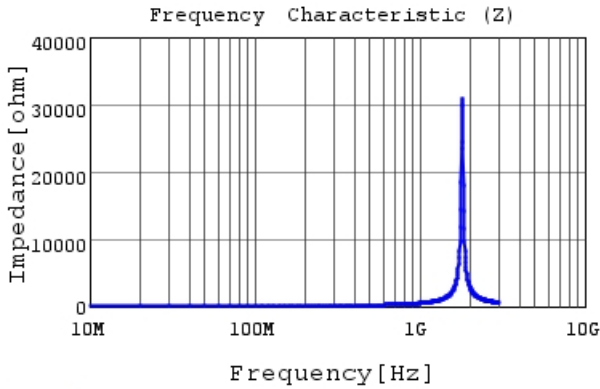
LQG15WH56NG02 |Z|
