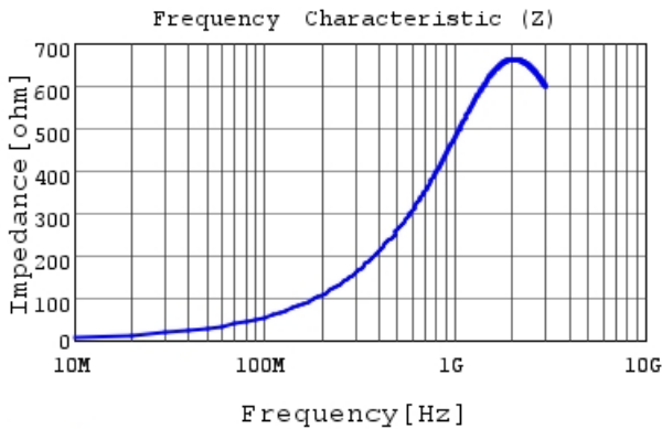
LQW18CNR10K00 |Z|
