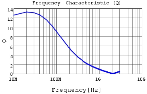
LQW18CNR10K00 Q
