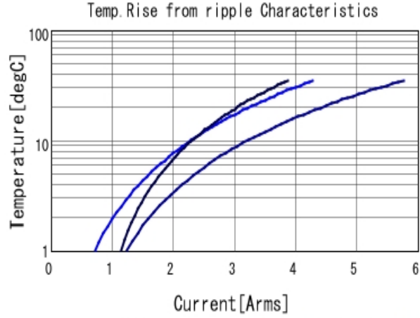
GCM32DC72A475KE02 Temp. rise ■ 100kHz ■ 500kHz ■ 1MHz
