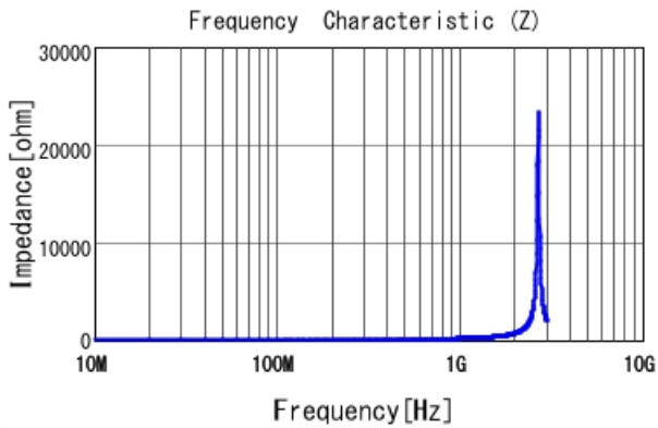
LQG15WH27NJ02 |Z|
