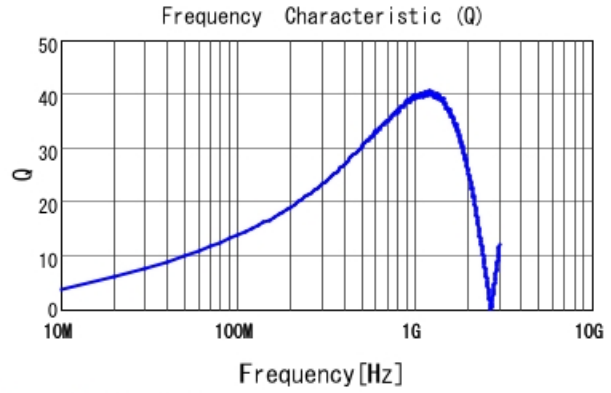
LQG15WH27NJ02 Q
