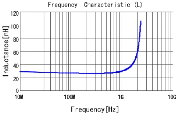
LQG15WH27NJ02 L
