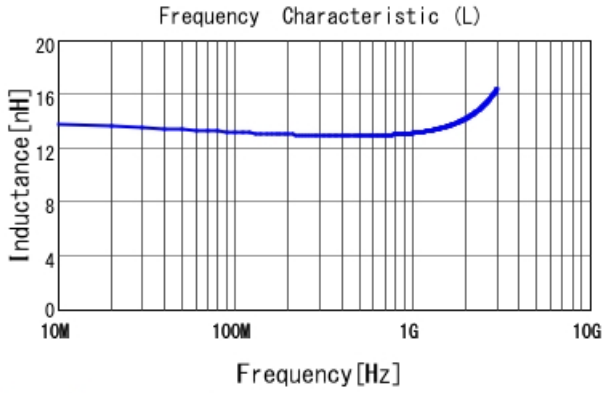
LQW15AN13NH0Z L
