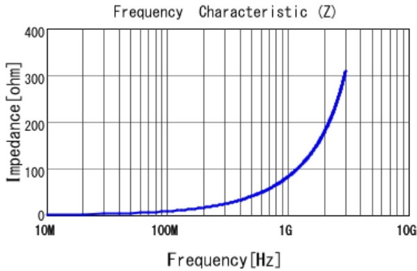
LQW15AN13NH0Z |Z|
