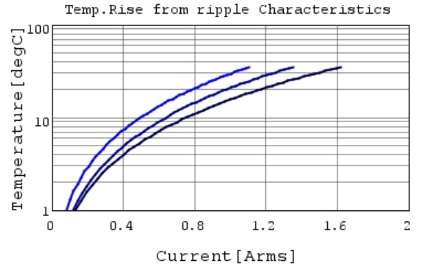
GRT155C81E224KE01 Temp.rise — 300kHz —
