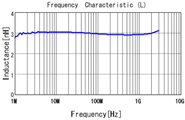
LQW15AN3N0G80 L
