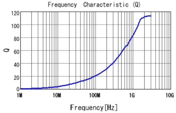
LQW15AN3N0G80 Q
