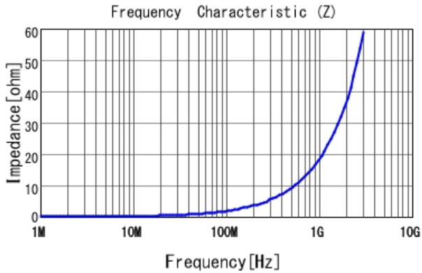
LQW15AN3N0G80 |Z|
