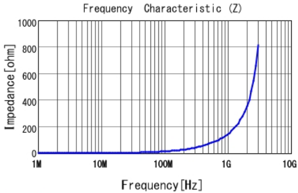
LQW18AN22NG8Z |Z|
