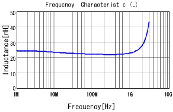
LQW18AN22NG8Z L
