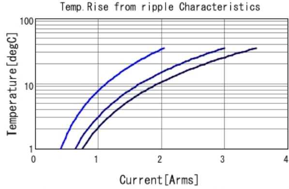
GRM31MR72A474KA35 Temp. rise — 200kHz — 500
