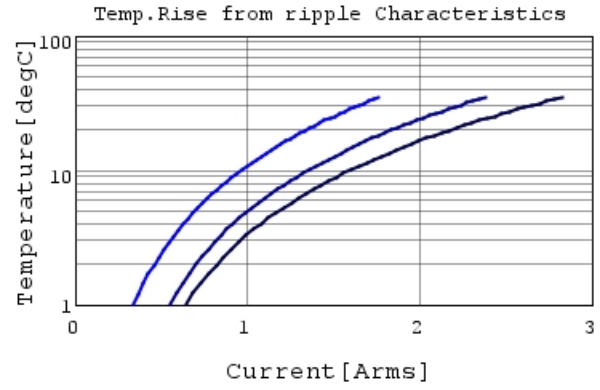
LLL185R71A224MA01 Temp.rise — 300kHz
