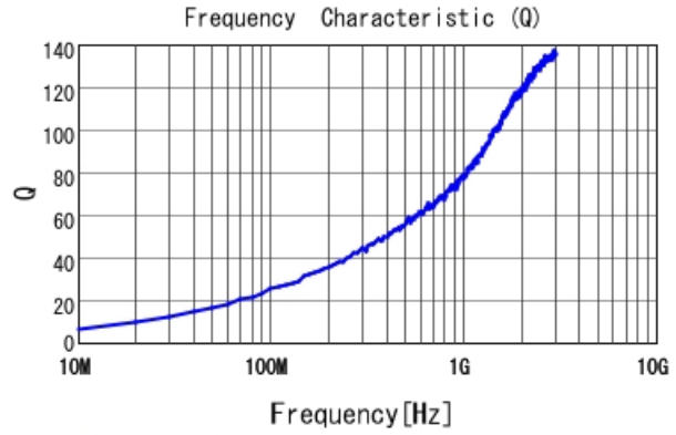
LQW15AN2N2C10 Q
