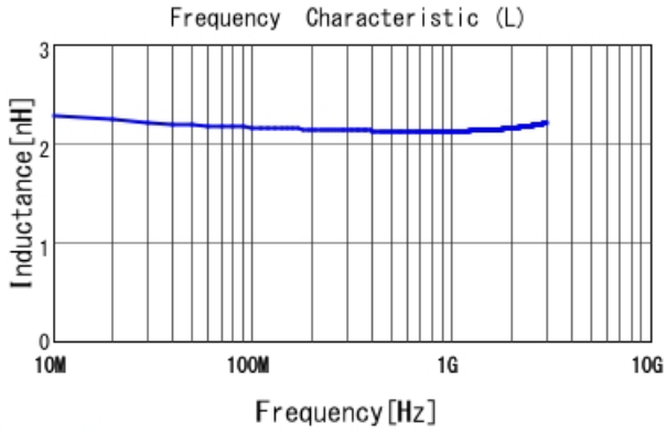
LQW15AN2N2C10 L
