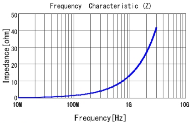
LQW15AN2N2C10 |Z|
