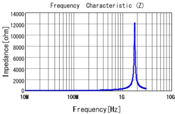
LQG15HH39NG02 |Z|
