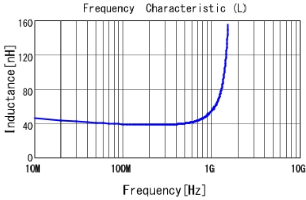
LQG15HH39NG02 L
