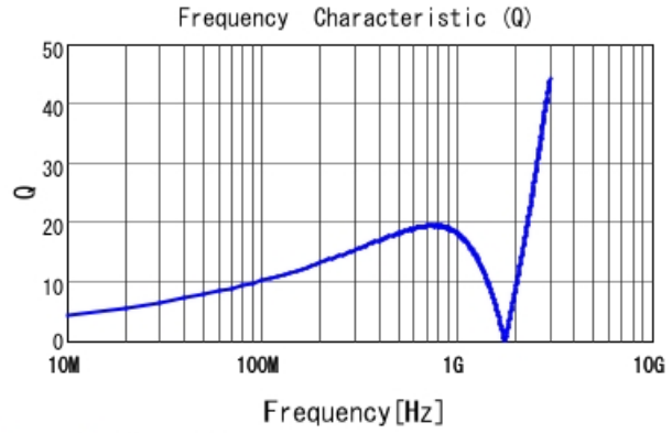
LQG15HH39NG02 Q
