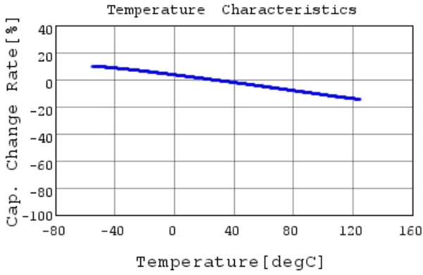
GA342DR7GF221KW02 C-Temp. capchange, DCOV, 1
