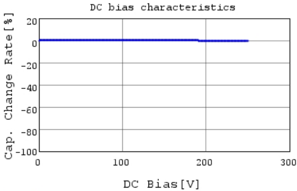
GA342DR7GF221KW02 C-DC bias capchange, 25.0c
