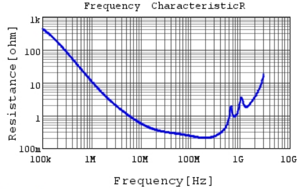
GA342DR7GF221KW02 R DCOV, 25degC
