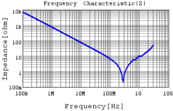
GA342DR7GF221KW02 |Z| DCOV, 25degC
