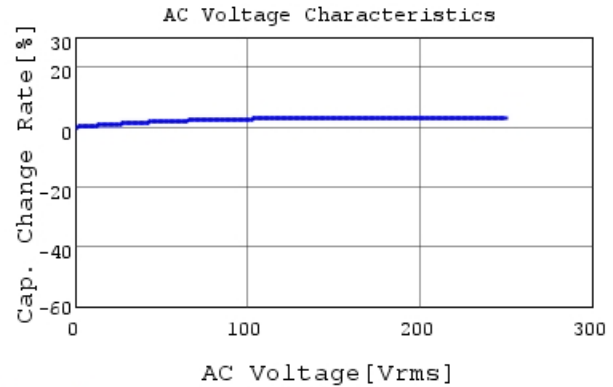
GA342DR7GF221KW02 C-AC Voltage capchange, DC
