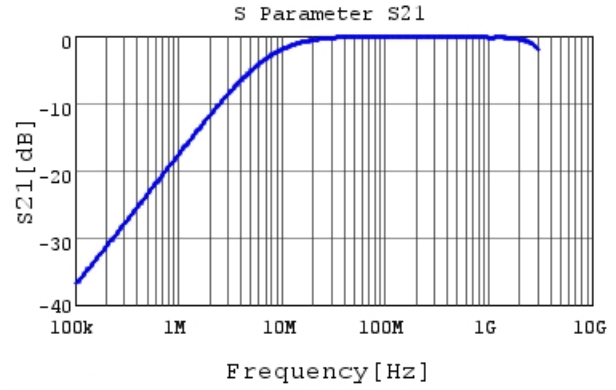
GA342DR7GF221KW02 S21 DCOV, 25degC
