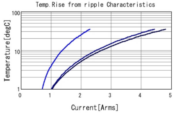
GRM31MR71C105MA01 Temp. rise — 100kHz — 500
