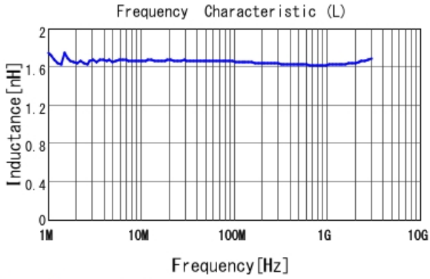
LQW15AN1N7D8Z L
