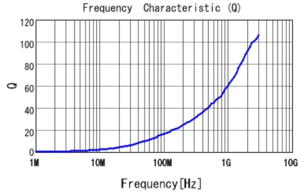
LQW15AN1N7D8Z Q
