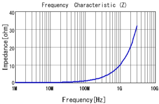
LQW15AN1N7D8Z |Z|
