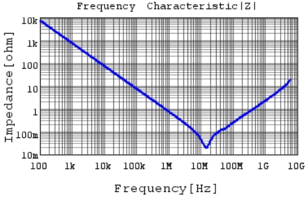
GCJ188R71E224KA12 |Z| DCOV,25degC
