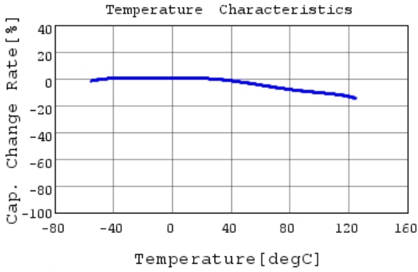
GCJ188R71E224KA12 C-Temp. capchange, DC0.0V,
