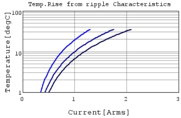
GCJ188R71E224KA12 Temp.rise — 300kHz —
