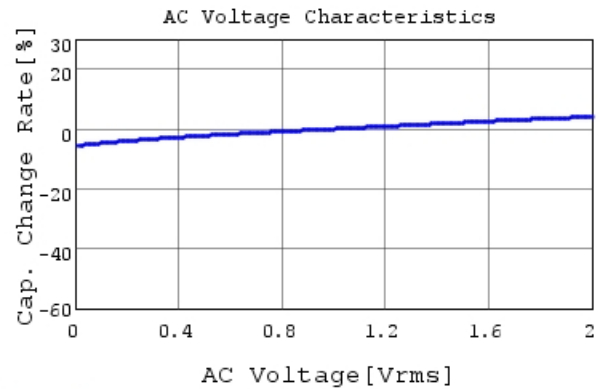
GCJ188R71E224KA12 C-AC Voltage capchange, Dc
