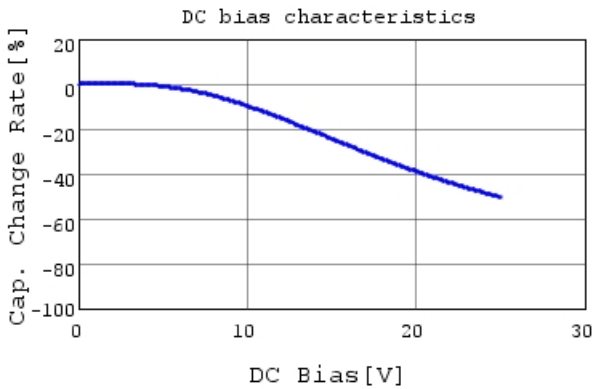
GCJ188R71E224KA12 C-DC bias capchange, 25.0c
