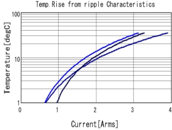
GRJ32DR72A225KE11 Temp. rise ■ 100kHz ■ 500kHz ■ 1MHz
