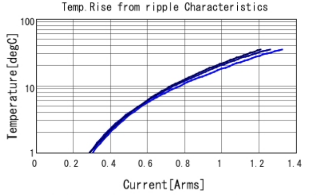
GQM2195C2E390JB12 Temp. rise — 500MHz — 700I
