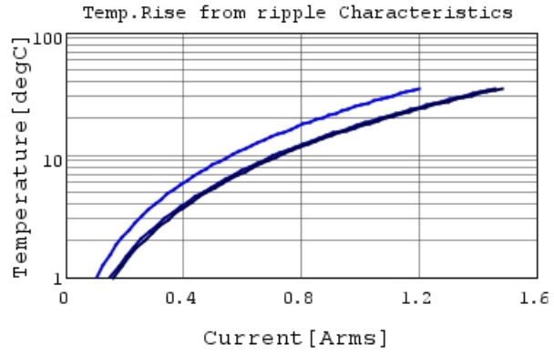
GCJ188R72A104KA01 Temp.rise — 400kHz —
