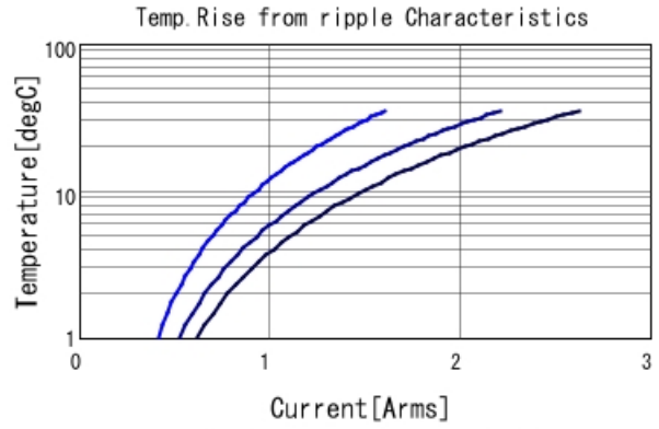
GCJ21BR71E274KA01 Temp. rise — 300kHz — 600
