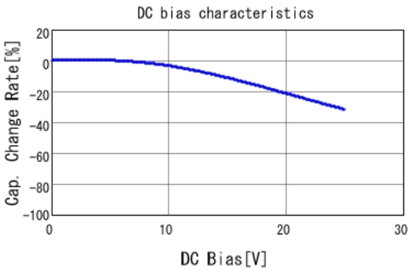
GCJ21BR71E274KA01 C-DC bias capchange, 25.0degC, A
