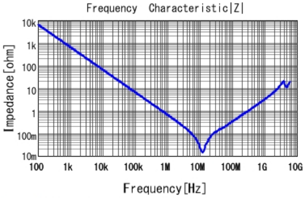
GCJ21BR71E274KA01 |Z| DCOV, 25degC
