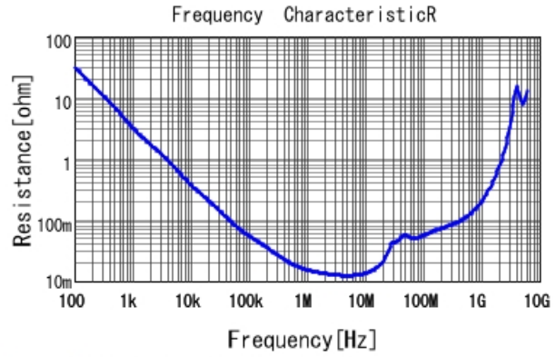
GCJ21BR71E274KA01 R DCOV, 25degC
